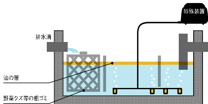
グリスアウト2号機 (エアーポンプタイプ)
